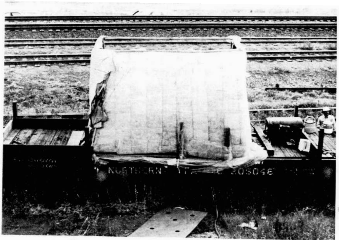
FIG. 3.5. LOAD CELL BARRIER.
