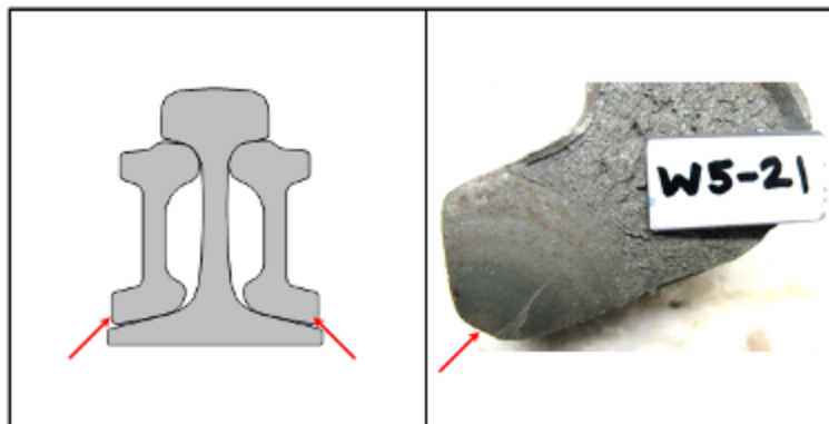
Figure 4. Bottom Edge Crack
