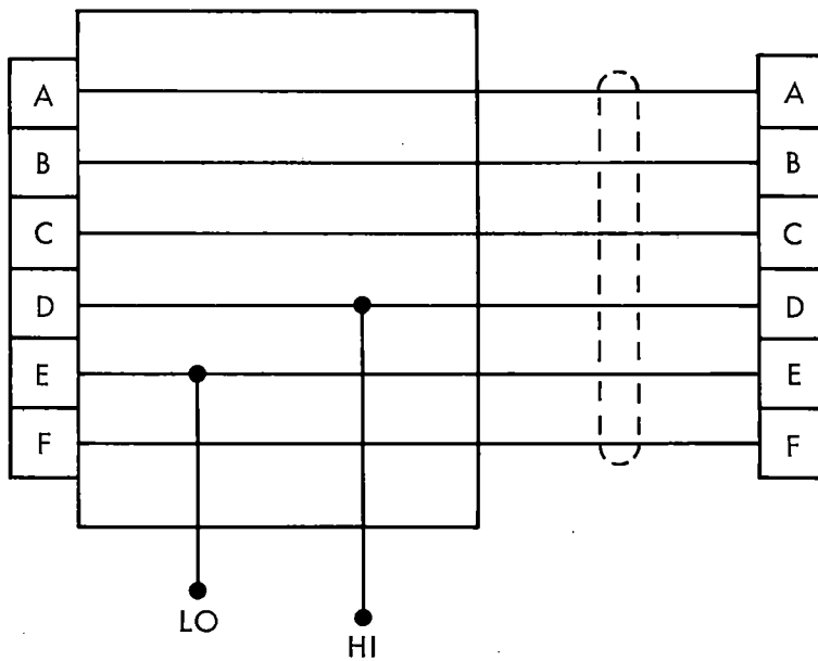
FIGURE A3-9. ALD CAL BOX
